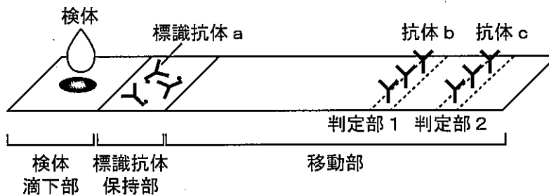
図1 ウイルス抗原の有無を判定する検査装置
